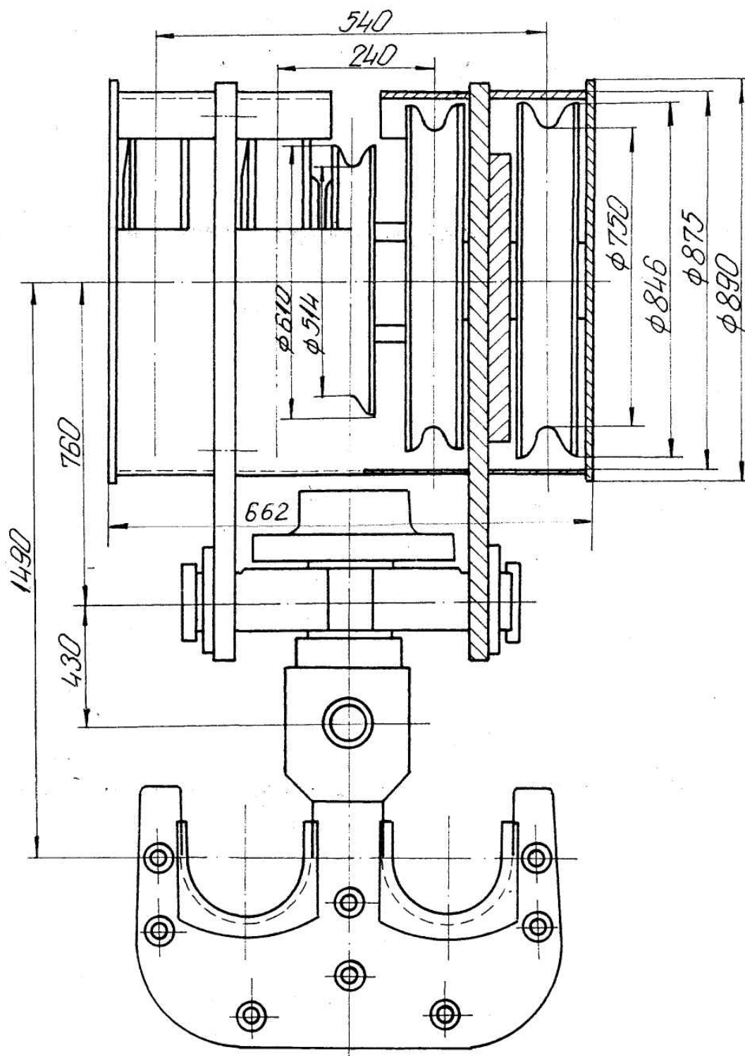
КУКА ПЛАСТИНЧАТА ДВУРОГА С РОЛКИ 500 kN
